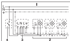
1. Lampe sans conducteur de neutre
