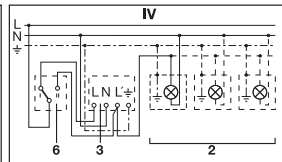
Anslutning via trappströmställare för permanent ljus resp. sensordrift Läge I: Sensordrift, av/på styrs av sensorn Läge II: Manuell drift, permanent belysning Observera: Frånkoppling av anläggningen är inte möjlig, man kan endast välja mellan läge I och läge II.
