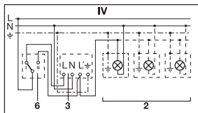
4. Allacciamento mediante deviatore per funzionamento automatico e in automatico
