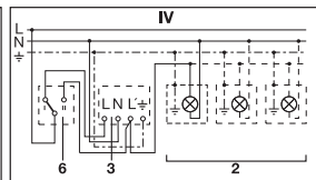
4. Aansluiting via een wisselchakelaar voor permanente verlichting en automatische werking
