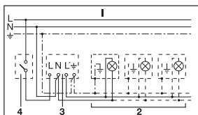
1. Lampada senza filo neutro
