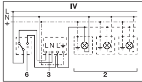
4. Sürekli ışık ve otomatik işletme için olan vaviyen şalter üzerinden olan bağlantı
