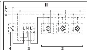
2. Nollajohdinhin suoraan valaisimelle
