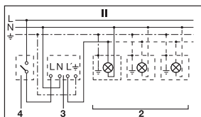
2. Lampada con presenza di filo neutro
