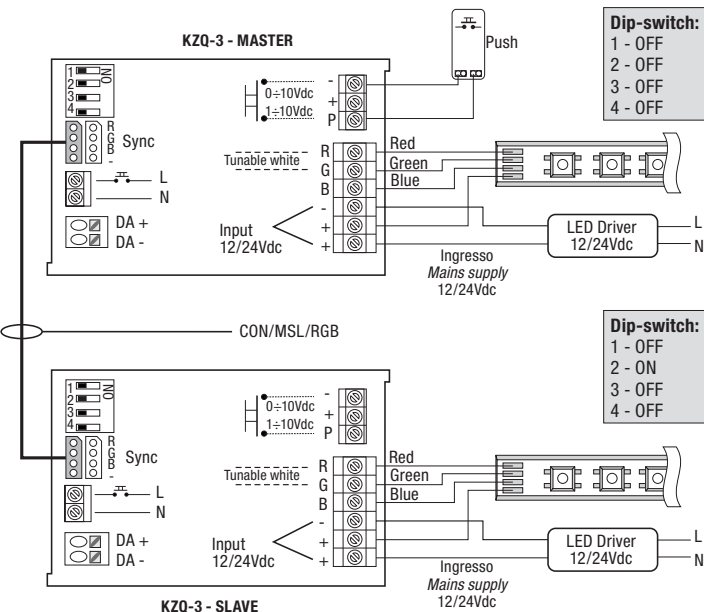
Fig. 7 - Comando sincronizzato con pulsante isolato - Synchronizd control with isolated button - Commande synchronisée avec bouton isolé - Synchronisierte Steuerung mit isoliertem Schalter
