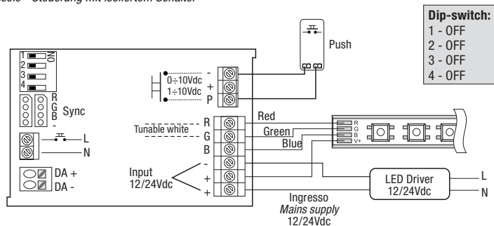
Fig. 1 - Comando con pulsante isolato - Command with isolated button - Commande avec bouton isolé - Steuerung mit isoliertem Schalter
