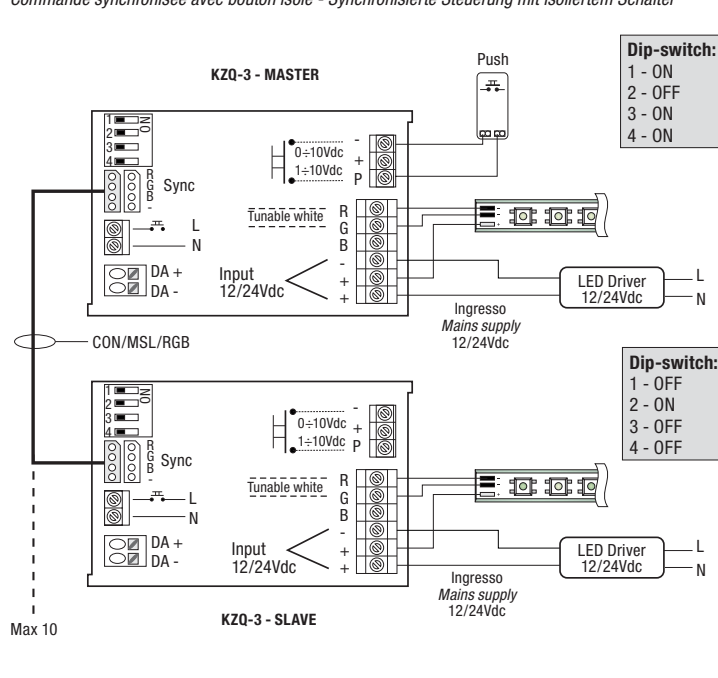
Fig. 18 - Comando sincronizzato con pulsante isolato - Synchronizd control with isolated button Commande synchronisée avec bouton isolé - Synchronisierte Steuerung mit isoliertem Schalter
