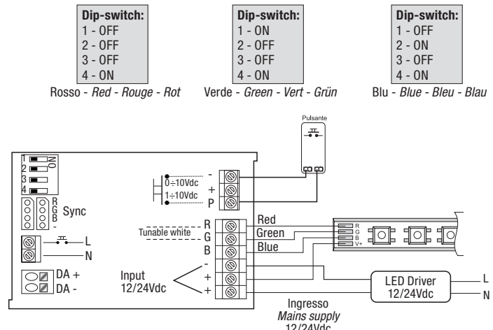
Fig. 5 - Regolazione colori singoli - Single color adjustment - Ajustement de couleur unique - Einfarbige Anpassung
