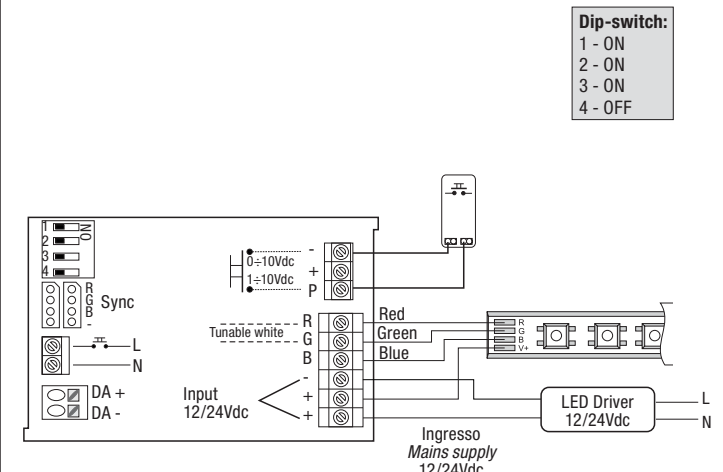
Fig. 6 - Sequenza colori fissi - Fixed color sequence - Séquence de couleurs fixe - Feste Farbfolge
