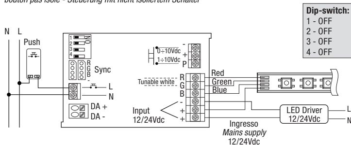
Fig. 2 - Comando con pulsante non isolato - Command with not isolated button - Commande avec bouton pas isolé - Steuerung mit nicht isoliertem Schalter
