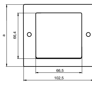
AQUADESIGN-Steckdose
